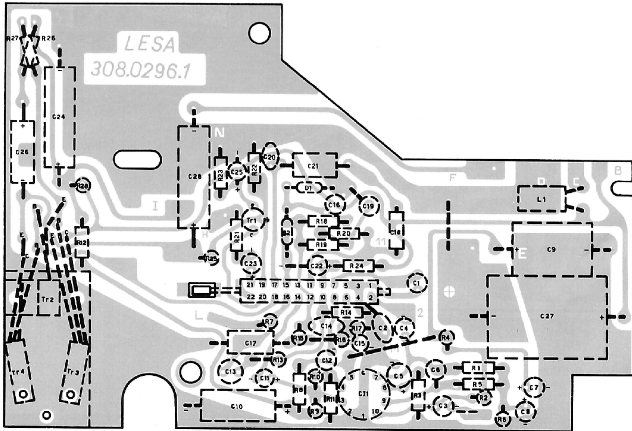
Circuito stampato amplificatore Renas LC 2
